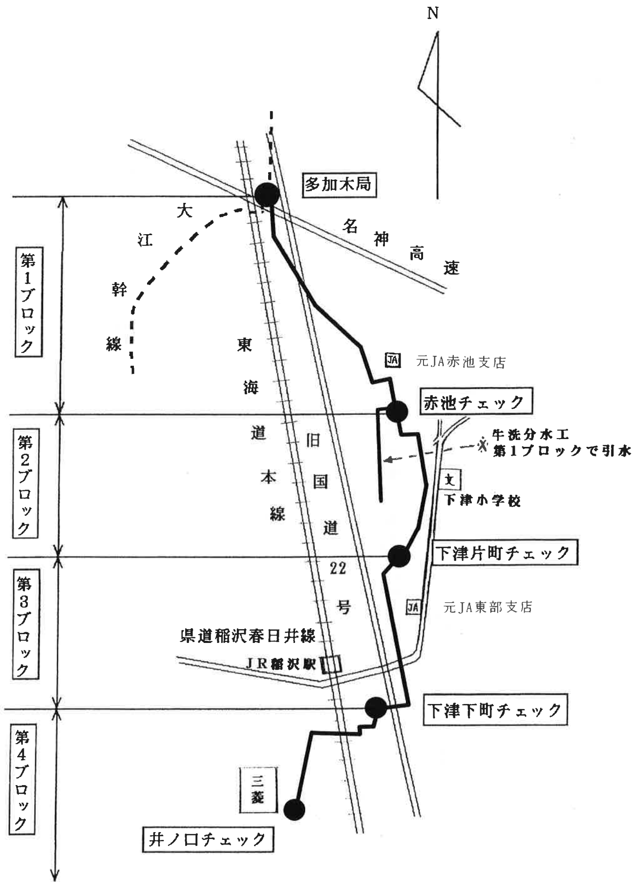
配水ブロック割図
